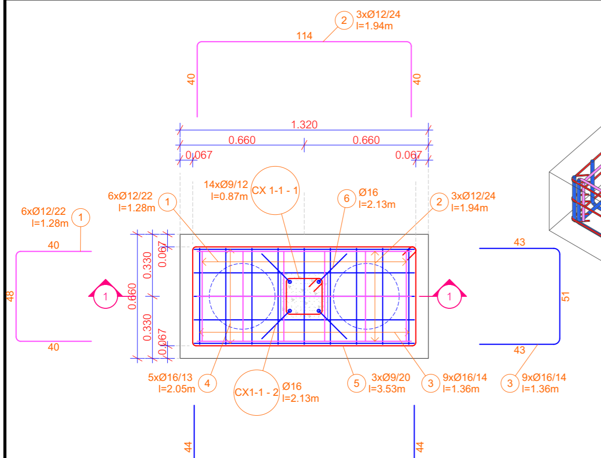
แบบขยายฐานราก F2 มาตรฐาน 1:20
