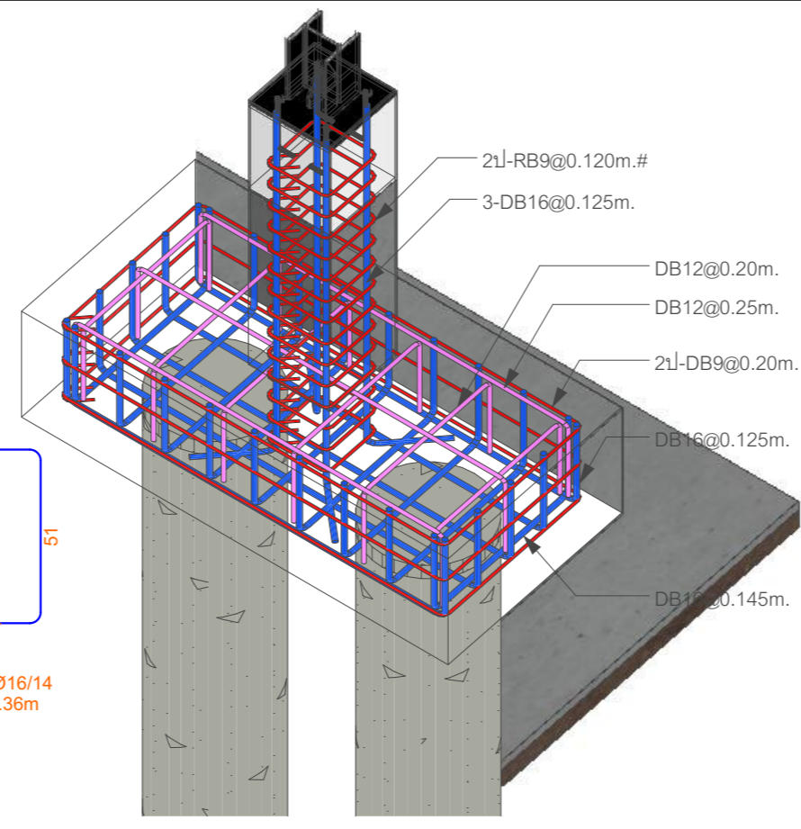
3D DETAIL F2 มาตรฐาน 1:20
